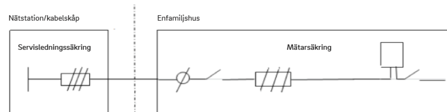
Figur 7: Skiss på anläggning med en måtarplats
