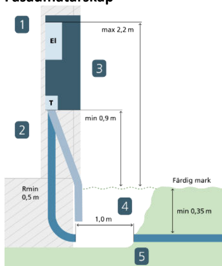
Figur 2. Montering av servisleddning och mätarskåp
