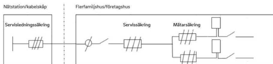
Figur 6: Skiss på anläggning med flera måtarplatser
